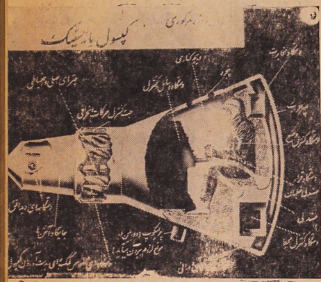
دستگاه های عمده سفینه فضائی طرح مرقوری در این گراور نشان داده میشود
